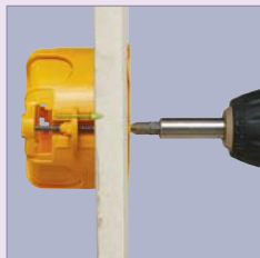
Gheare de fixare adaptate la grosimea peretelui. Poziționare automată, chiar și cu o șurubelniță electrică
