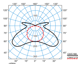
AragF 12 PXW 20-65/16ML-840 ET (stage 8)
