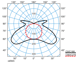
AragF 12 PXW 20-65/16ML-840 ET (stage 11)
