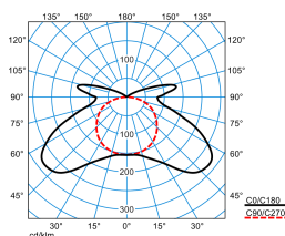
AragF 12 PXW 20-65/16ML-840 ET (stage 15)
