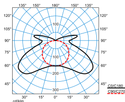
AragF 12 PXW 20-65/16ML-840 ET (stage 14)
