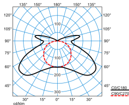
AragF 12 PXW 20-65/16ML-840 ET (stage 13)
