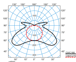
AragF 12 PXW 20-65/16ML-840 ET (stage 3)
