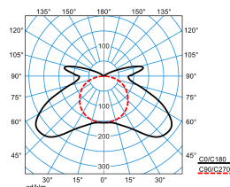
AragF 12 PXW 20-65/16ML-840 ET (stage 4)
