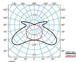
AragF 12 PXW 20-65/16ML-840 ET (stage 6)
